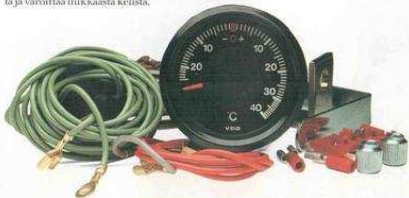
Kelivaroitin mittaa lämpötilan tienpinnan yläpuolelta ja varoittaa liukkaasta kelistä.
